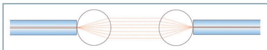
1 Grafische Darstellung der Funktionsweise eines Linsensteckers
