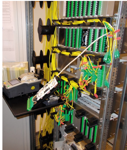
Bild 2: Auf dem Spleißtisch des Rack-Systems kann der Netztechniker das Spleißgerät abstellen und es nahe an der Baugruppe betreiben
