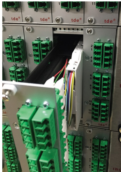
Bild 3: Auf 46 Höheneinheiten können Netzwerktechniker mit tDF bis zu 4032 Fasern mit LC-Steckverbindern terminieren
