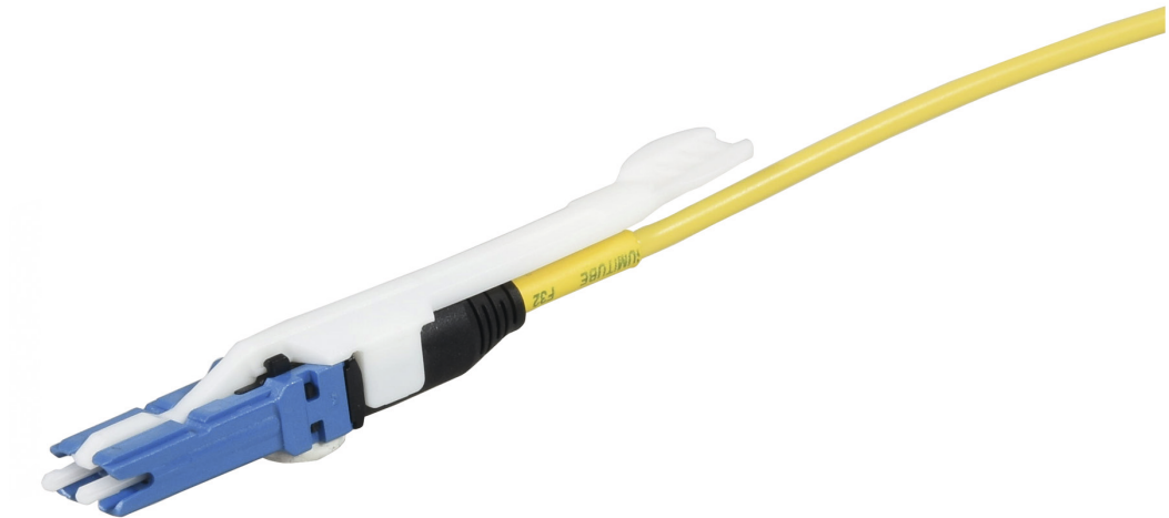
Bild 2. TDE Trans Data Elektronik hat die kompakte CS-Anschluss-technik bereits in seine tML-Systemplattform integriert. Im Rückraum setzen die Module auf die MPO-Technik und binden auf der Vorderseite CS-Steckverbinder ein. Auf diese Weise lassen sich bis zu 128 x 2 Fasern mit insgesamt 256 Fasern auf einer Höheneinheit realisieren.
