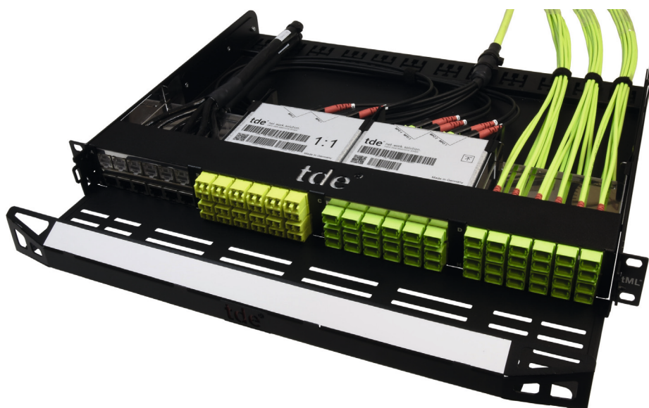
Bild 3. Skalierfähige Verkabelungssysteme wie das tML setzen auf den 12-, 24- oder 32-Faser-MPO im Rückraum und binden vorne bereits die im Gegensatz zum LC-Duplex-Steckverbinder deutlich kompakteren CS-Steckverbinder mit zwei Fasern oder auch die SN- sowie MDC-Steckverbinder mit jeweils zwei bis acht Fasern ein.
