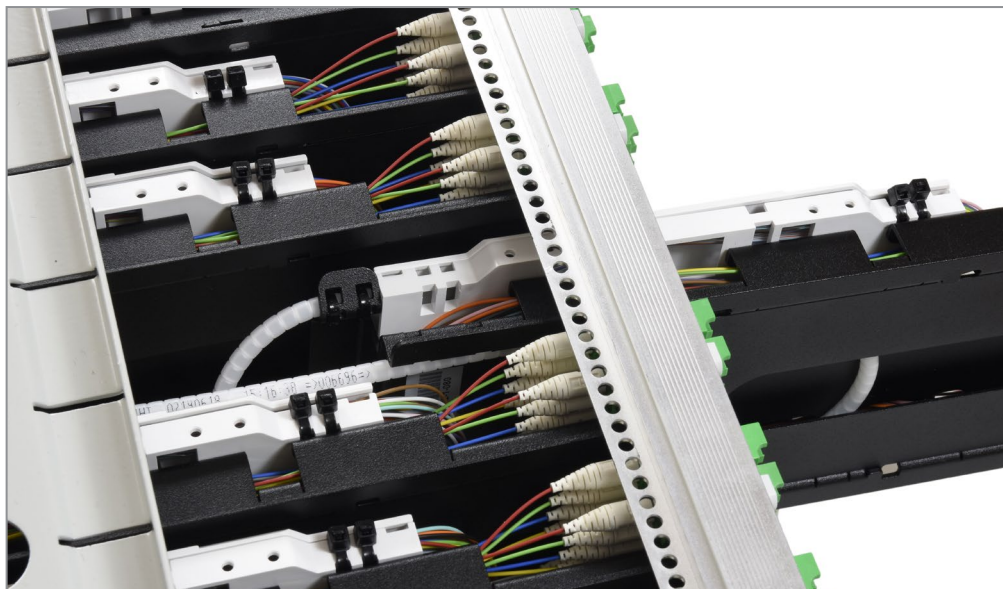
Integriertes Bündelader-Überlängenmanagement
